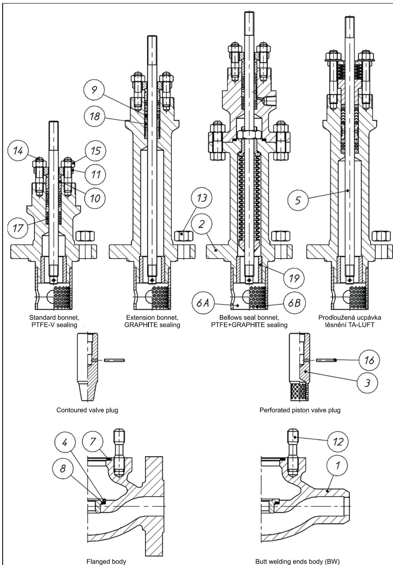
Fig. 1e. Control valve
